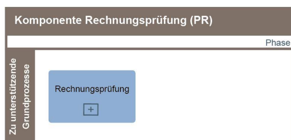
Abbildung 3.16: Komponente – Rechnungsprüfung
